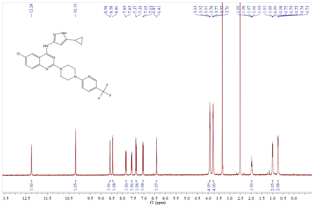
Compound 8e
