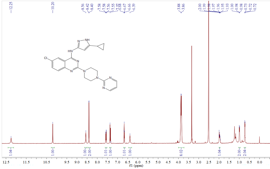
Compound 9a
