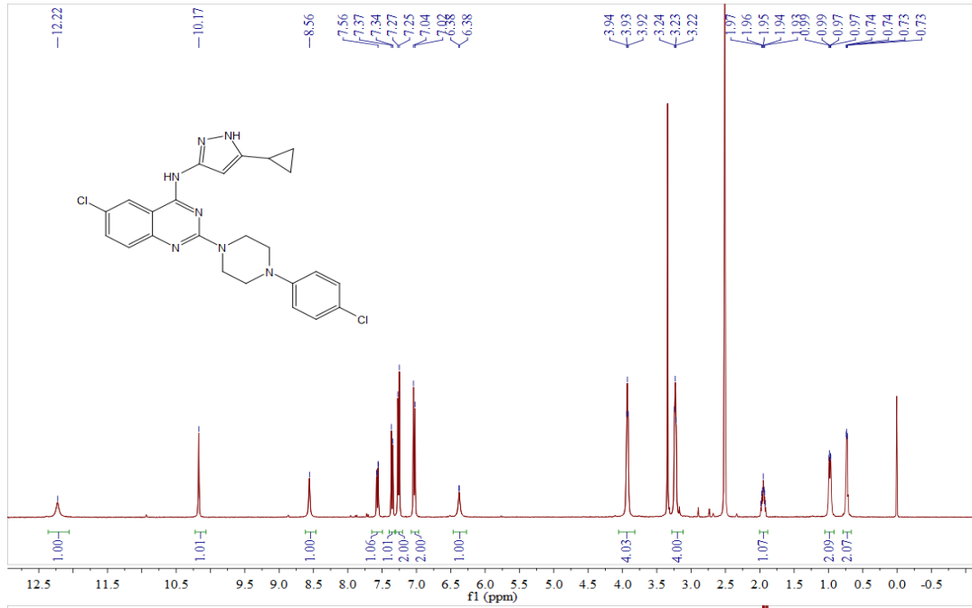
Compound 7e
