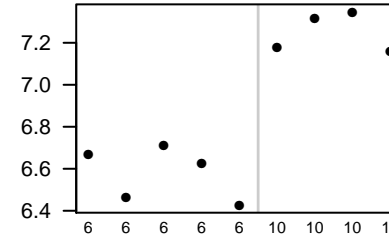
Sept4
