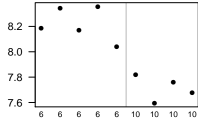
Sirt2
