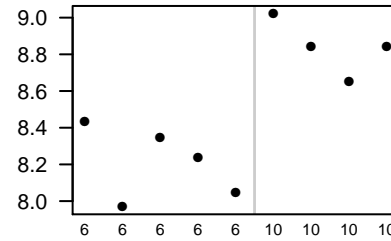
Plip
