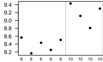
Ddx18
