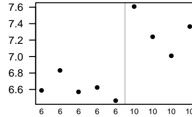
Kif11
