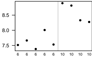
Dhcr24
