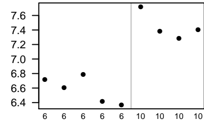
Mpz
