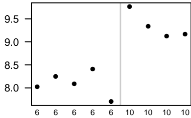
Fxyd1
