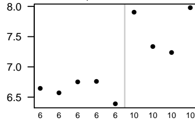
Spock1
