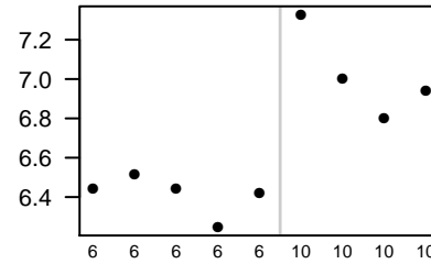
Npdc1
