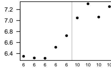
Dpysl4
