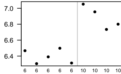
RGD735065
