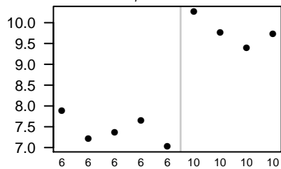
Scn7a
