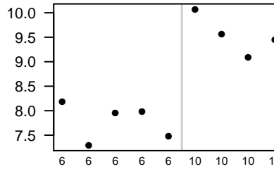
Tmem98
