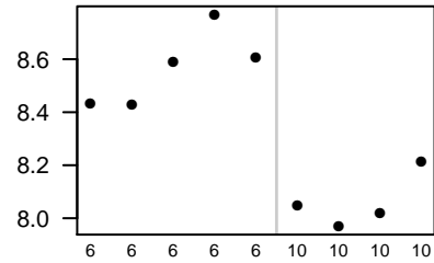
Nupr1
