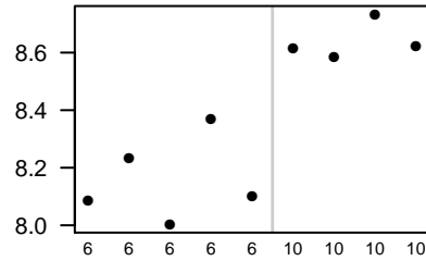
Chn2
