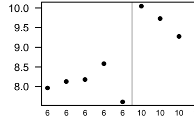
Rras2
