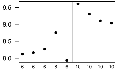
Prkcz
