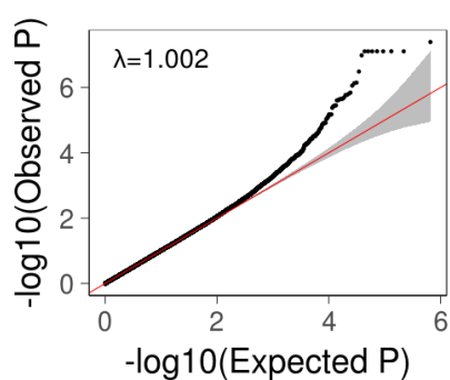
INDEL
