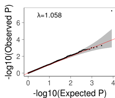
ORF
