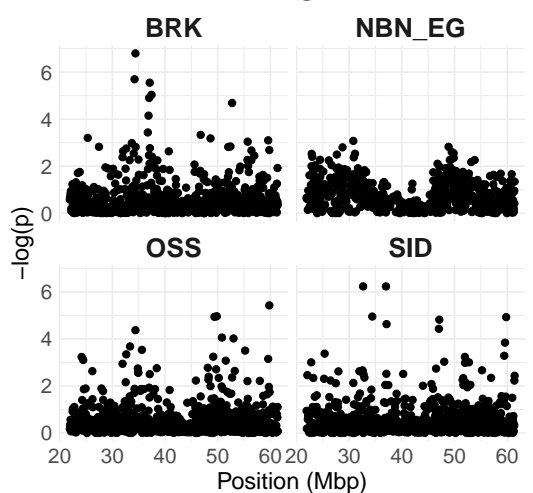
iHS
