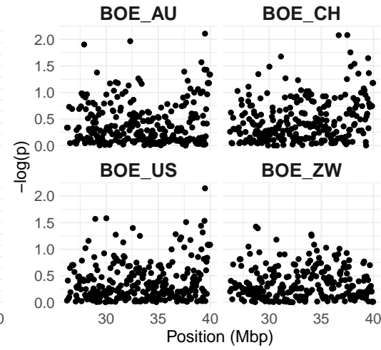
iHS
