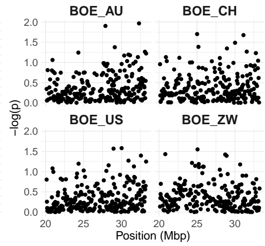
iHS
