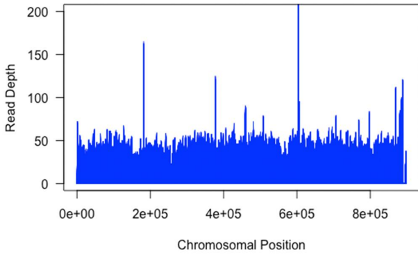
VL38 - chr25
