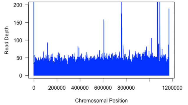
VL38 - chr28
