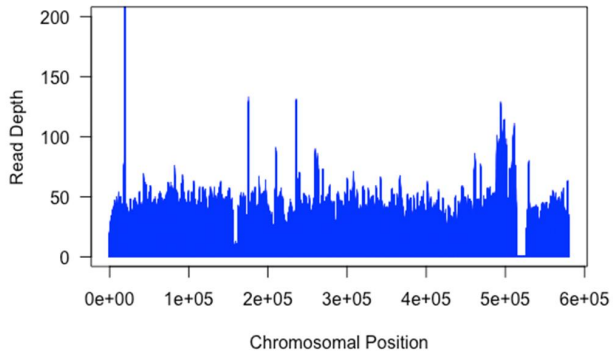
VL38 - chr11
