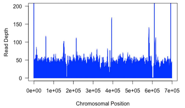
VL38 - chr16
