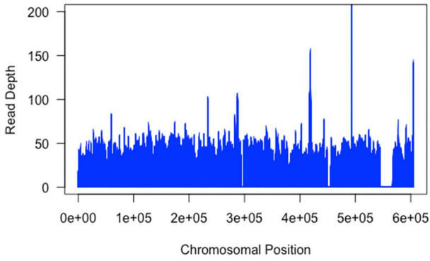
VL38 - chr7
