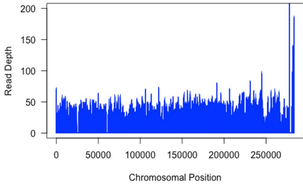
VL38 - chr1
