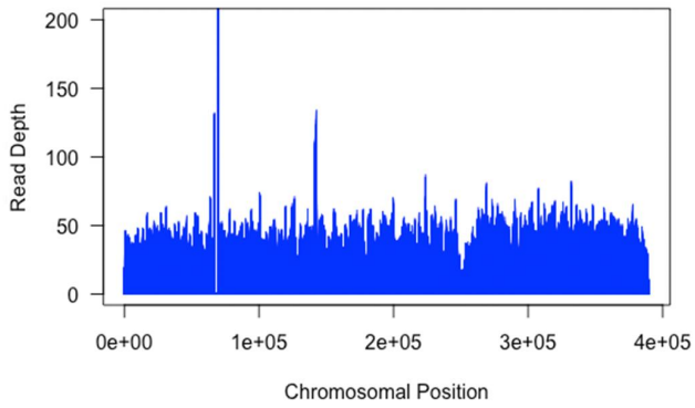
VL38 - chr3
