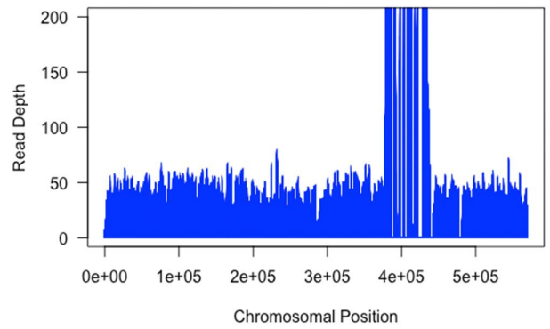
VL38 - chr12
