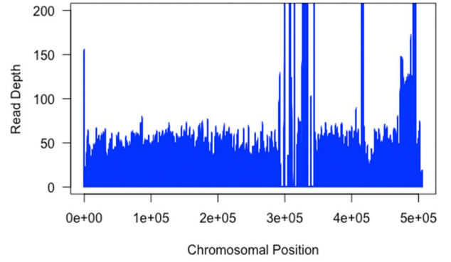
VL38 - chr8
