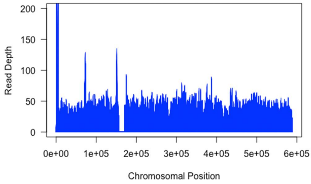
VL38 - chr9
