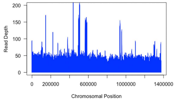
VL38 - chr30
