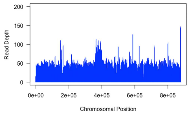
VL38 - chr24
