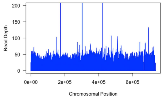
VL38 - chr18
