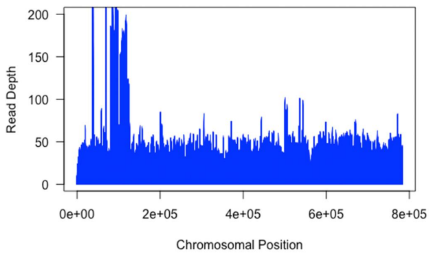
VL38 - chr23
