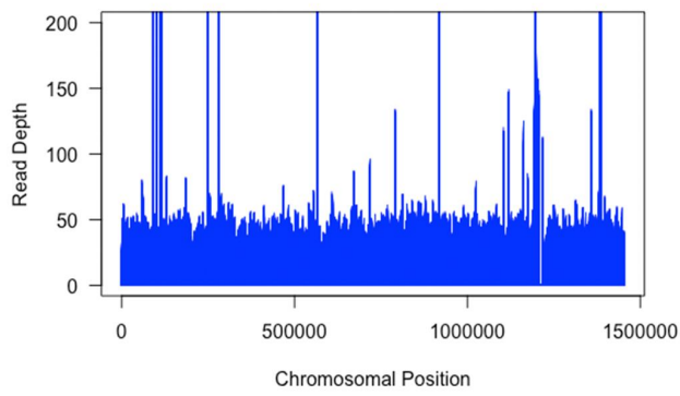
VL38 - chr33
