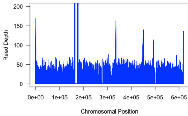
VL38 - chr15
