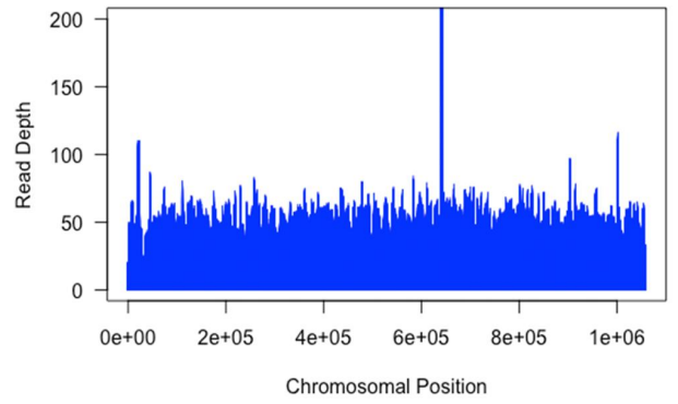
VL38 - chr26
