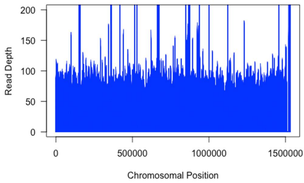
VL38 - chr31
