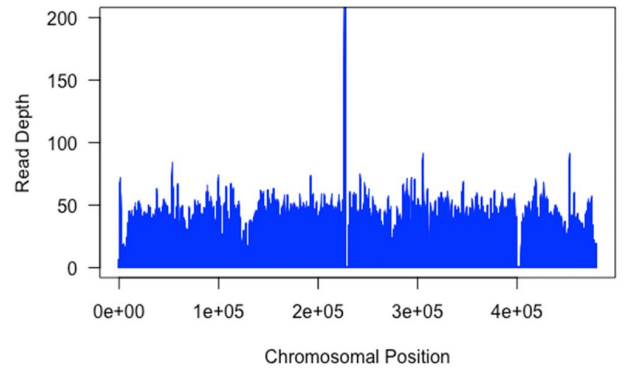
VL38 - chr4
