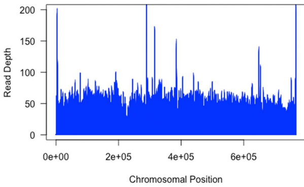
VL38 - chr21
