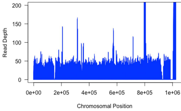
VL38 - chr27
