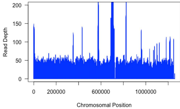
VL38 - chr29
