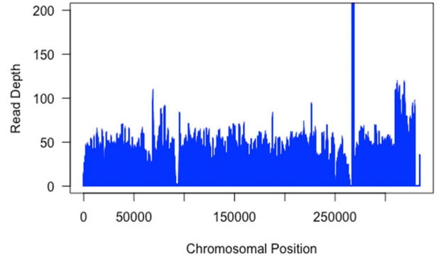
VL38 - chr2
