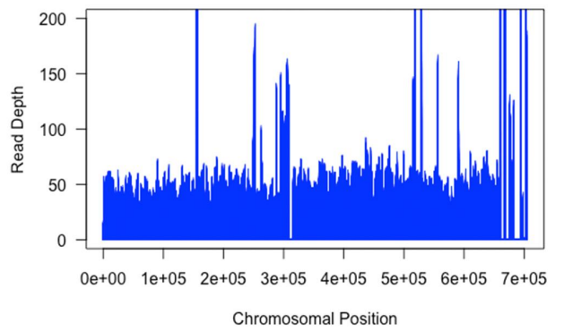
VL38 - chr22
