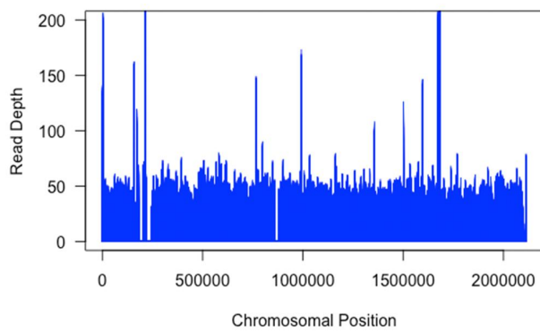
VL38 - chr35
