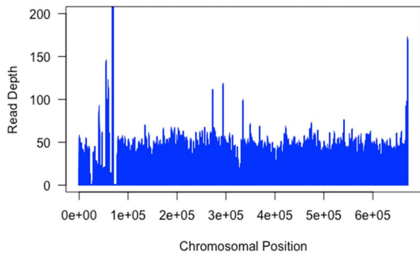
VL38 - chr17
