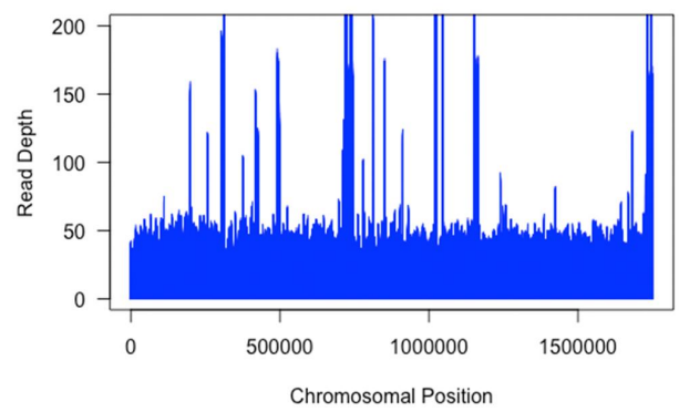
VL38 - chr34
