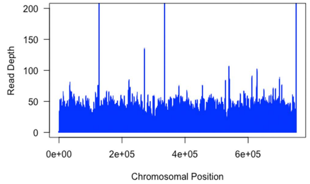
VL38 - chr20
