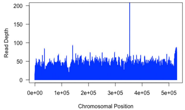
VL38 - chr6
