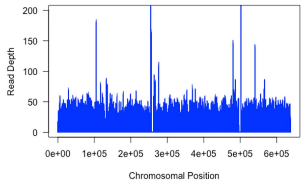
VL38 - chr14
