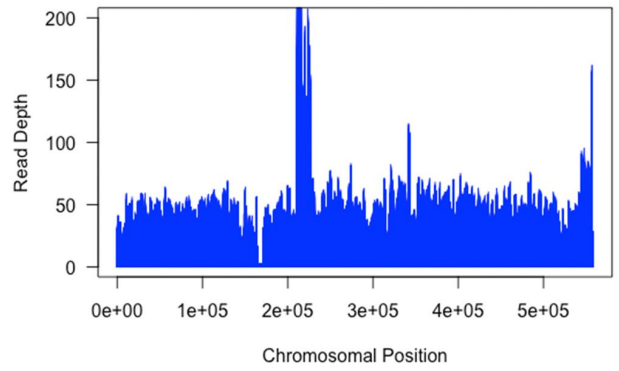
VL38 - chr10
