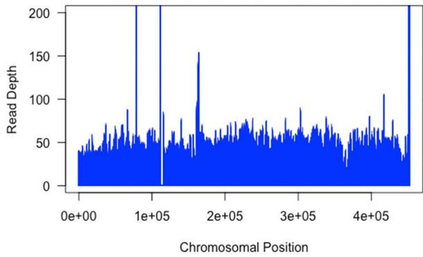
VL38 - chr5
