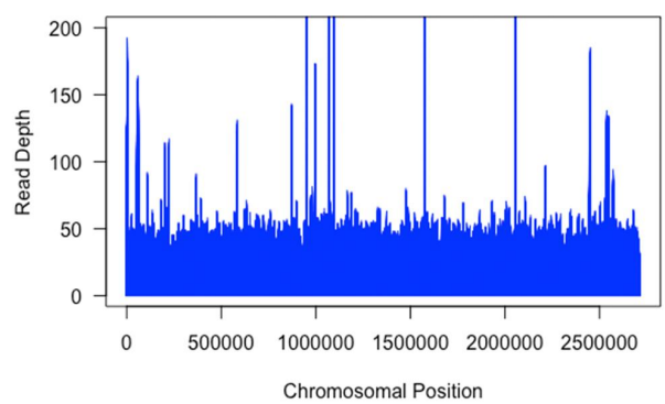
VL38 - chr36
