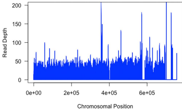
VL38 - chr19
