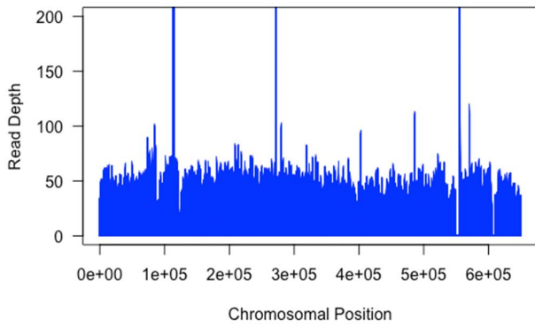
VL38 - chr13
