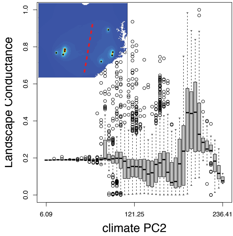
SNP dataset
