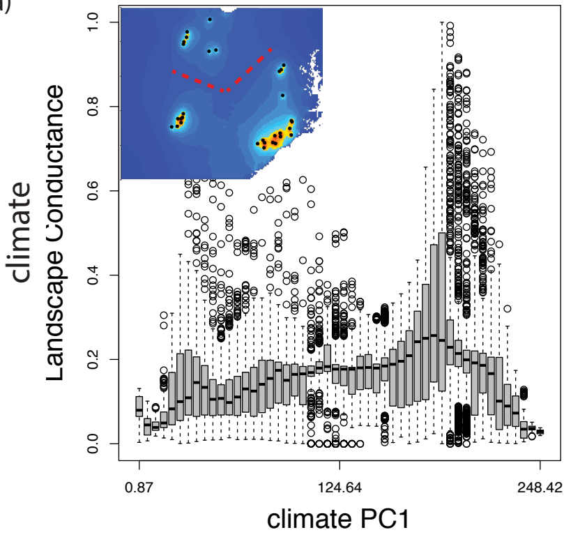
SSR dataset
