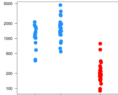
PF3D7_0422900
