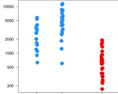
PF3D7_0501300
