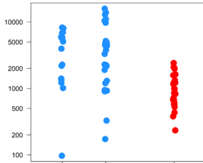
PF3D7_0420300
