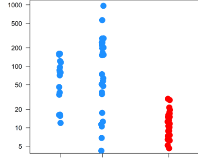
PF3D7_0522300
