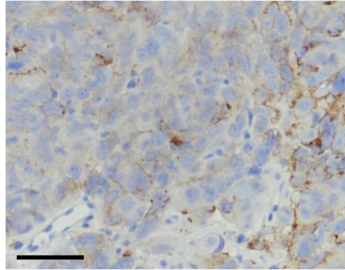
HER2
