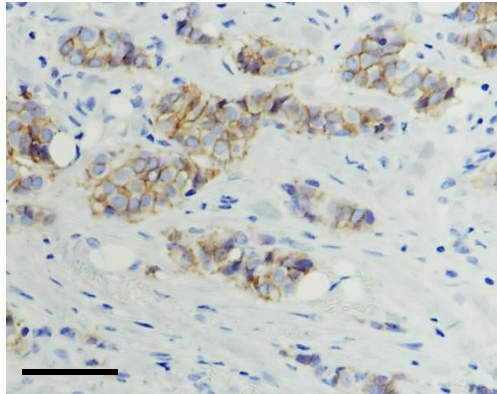
HER2
