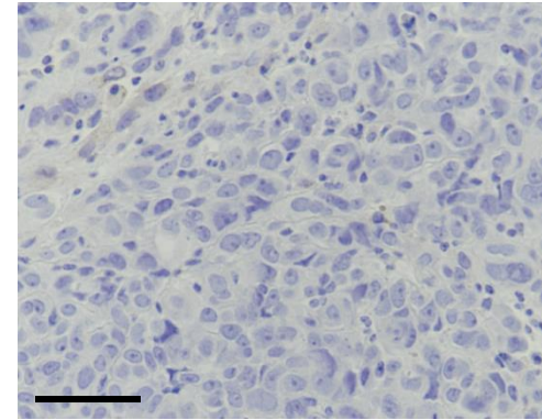
EGFR
