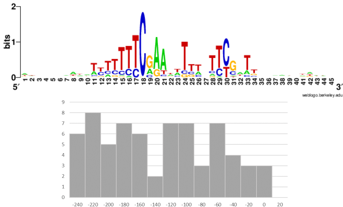
Motif #9 (68 sites)
