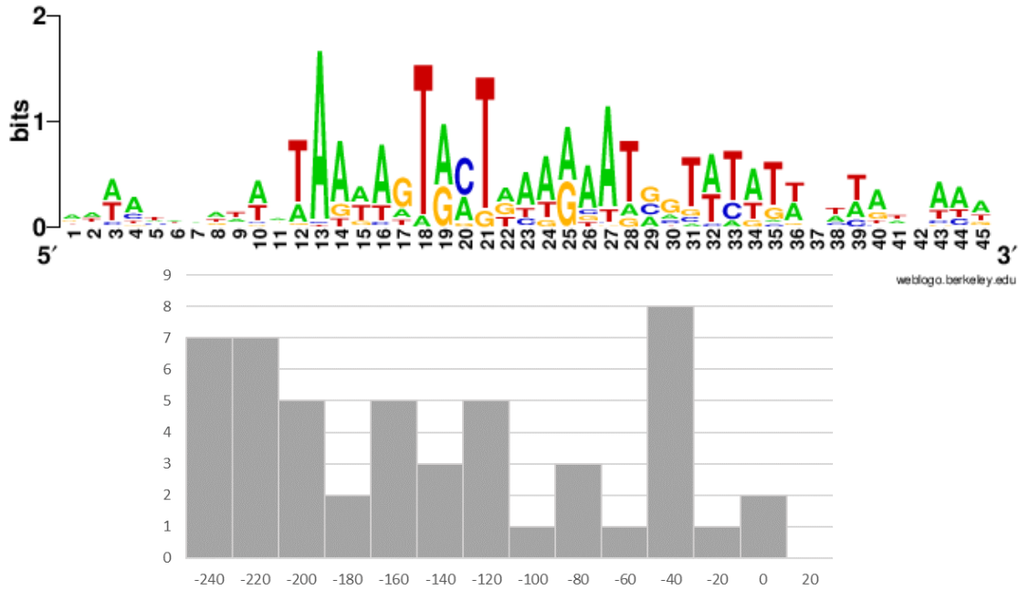
Motif #5 (50 sites)
