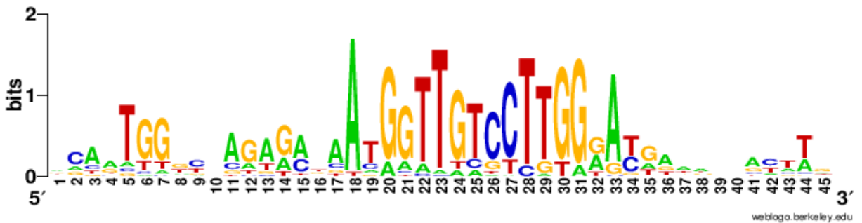
Motif #2 (50 sites)
