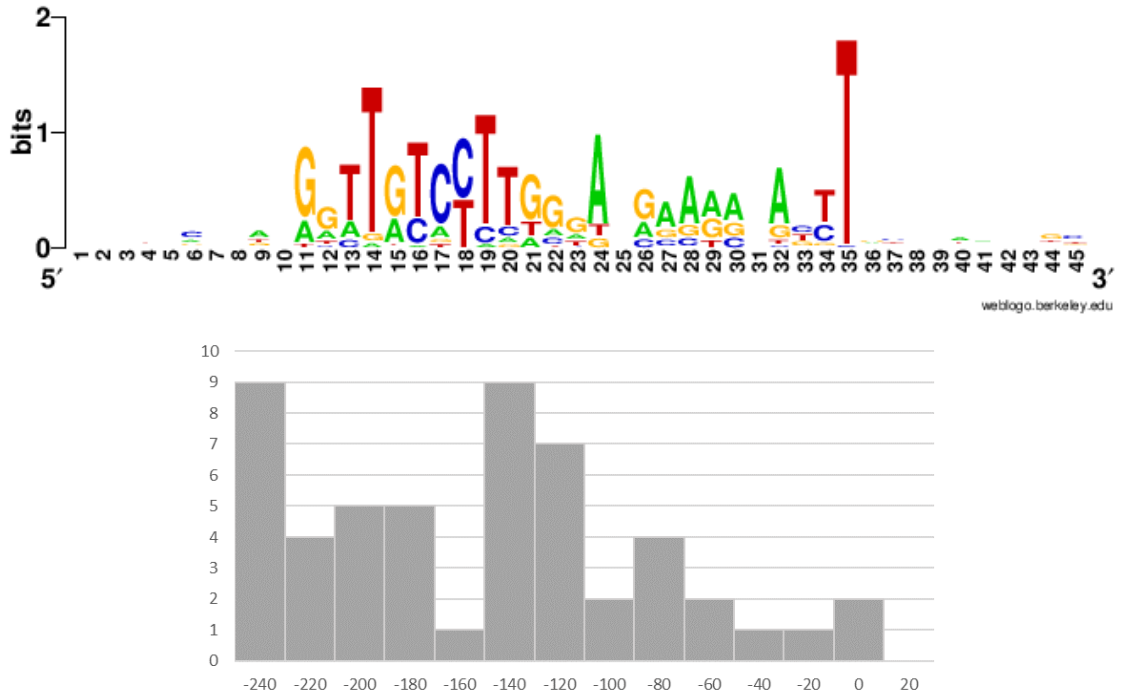
Motif #8 (52 sites)
