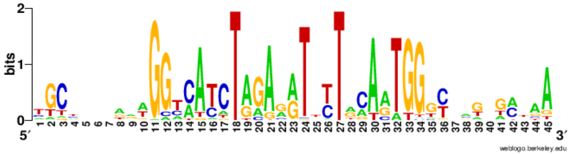
Motif #1 (50 sites)
