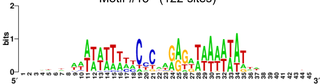
Motif #15 (122 sites)
