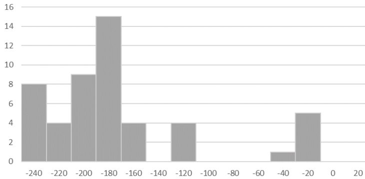
Motif #2 (50 sites)
