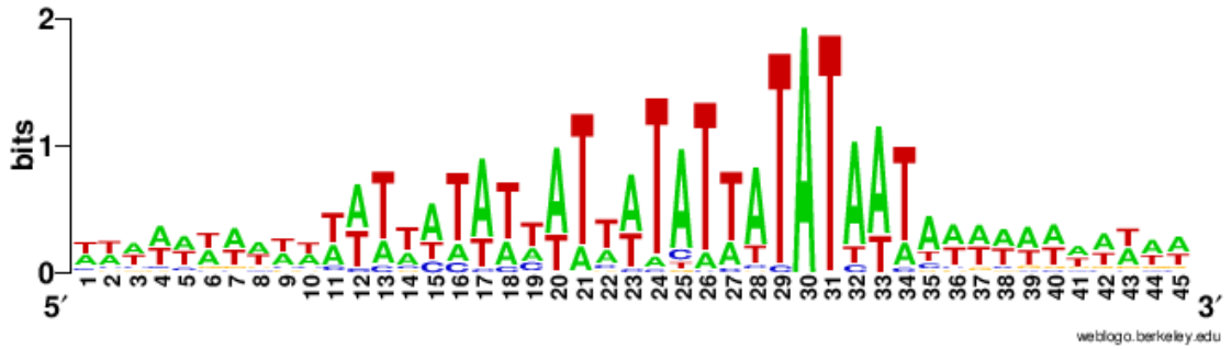
Motif #5 (264 sites)
