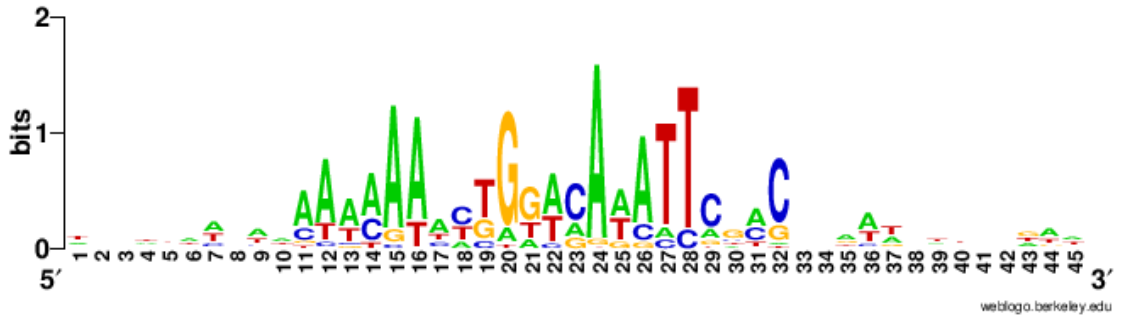
Motif #3 (70 sites)
