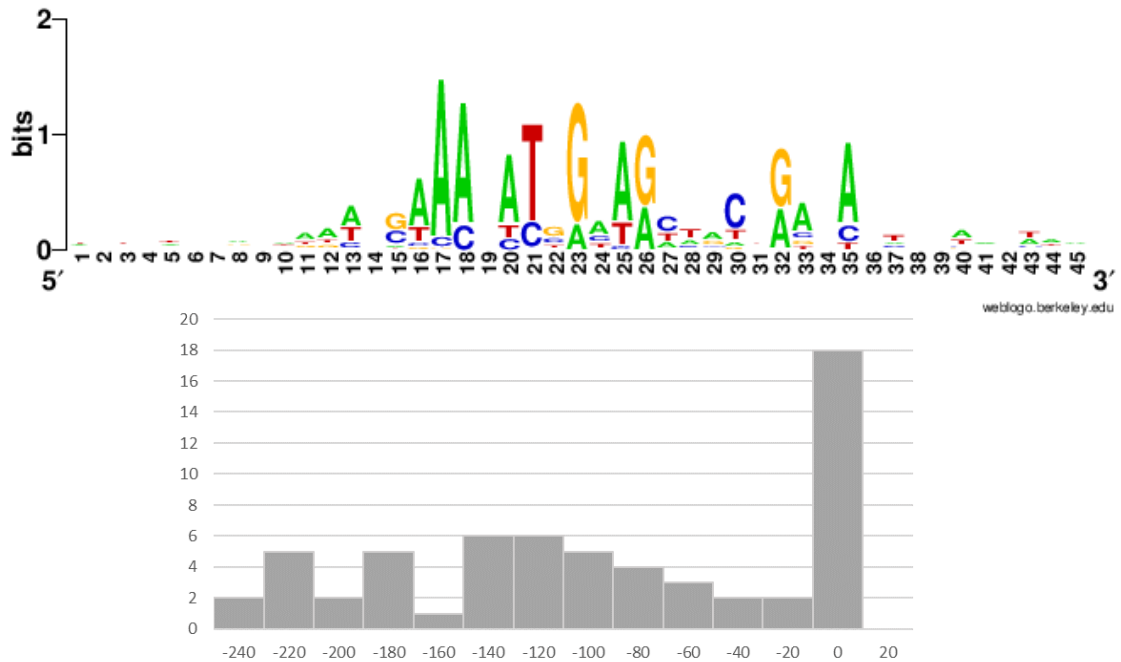
Motif #2 (61 sites)
