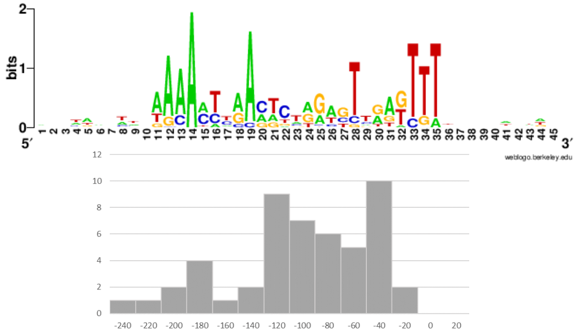
Motif #1 (50 sites)
