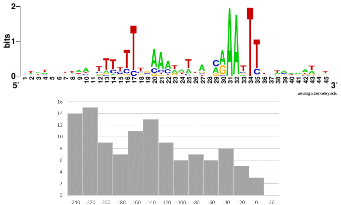
Motif #8 (113 sites)
