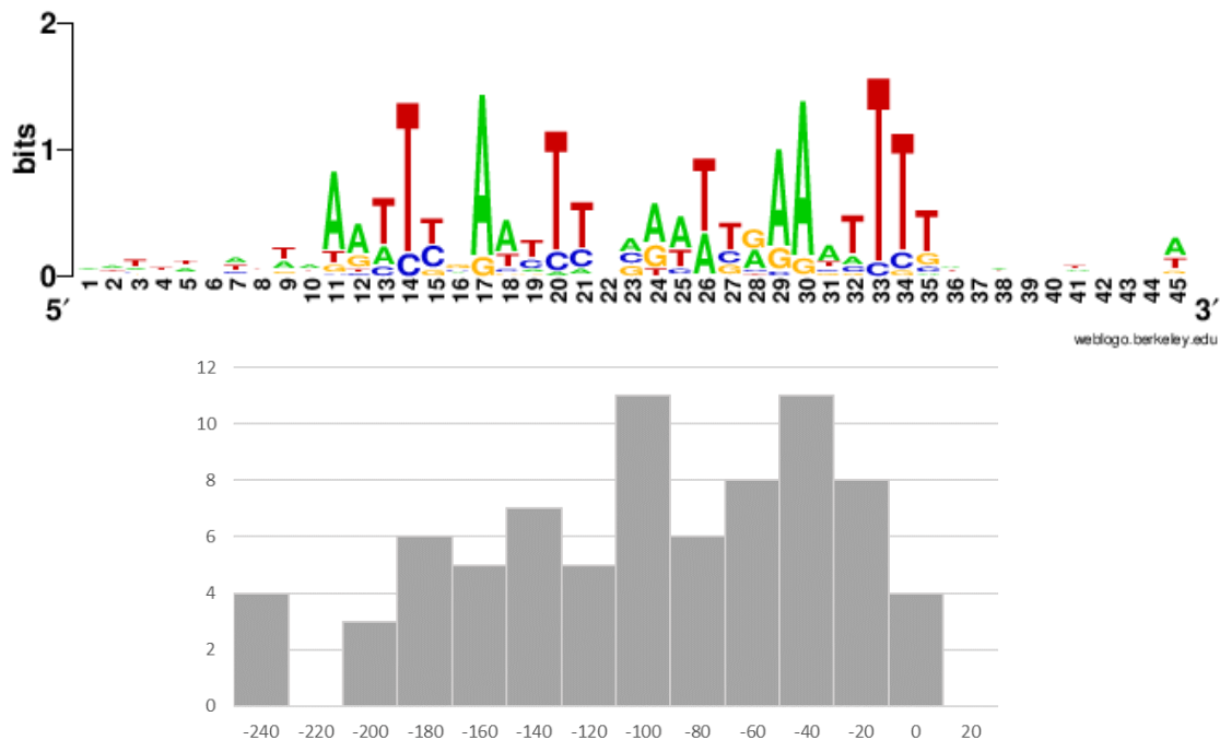
Motif #10 (78 sites)
