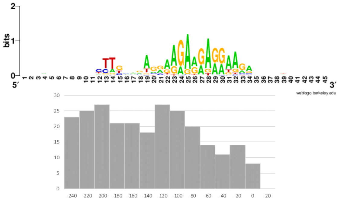
Motif #6 (254 sites)
