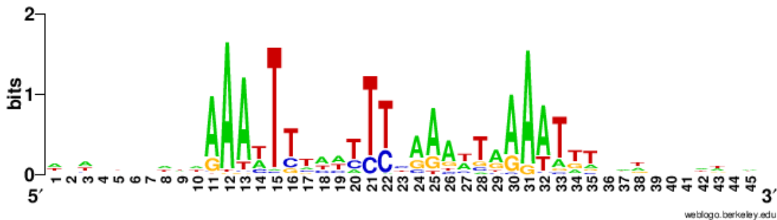
Motif #13 (128 sites)
