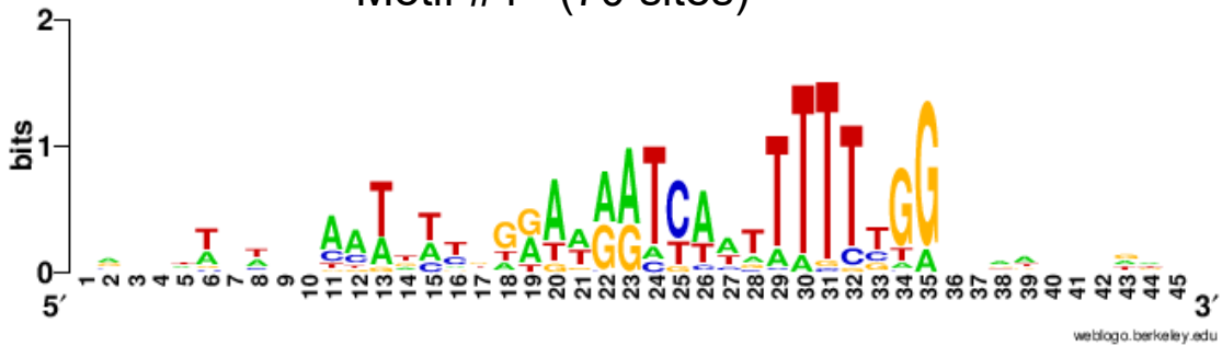
Motif #4 (70 sites)
