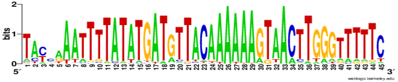
Motif #5 (50 sites)
