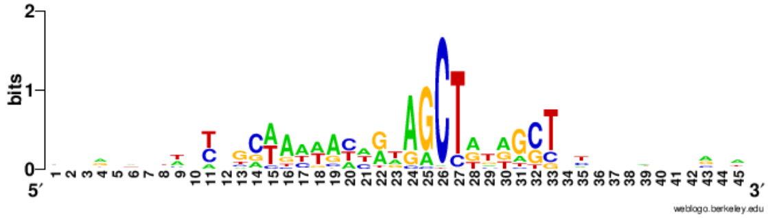
Motif #5 (52 sites)
