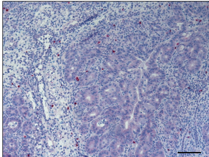
C. jejuni WT
