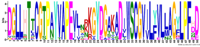
Motif 1
