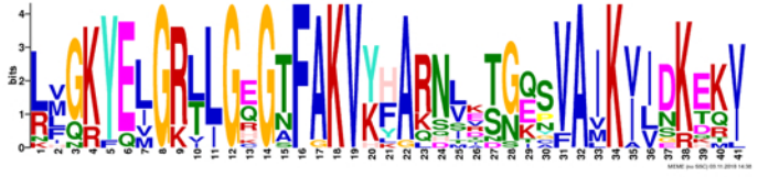
Motif 5
