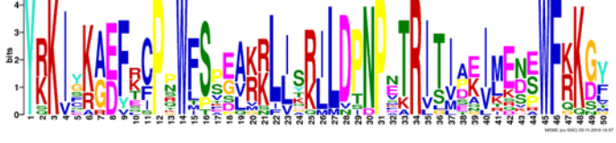
Motif 3
