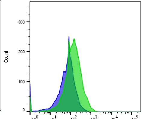
CD105
