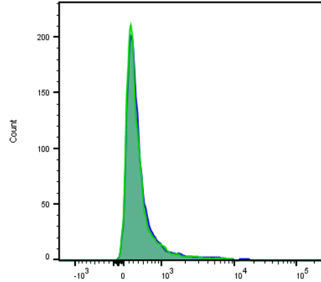
CD34
