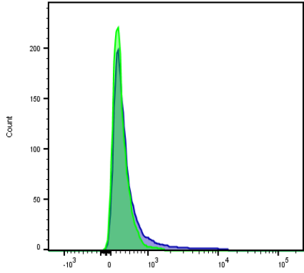
CD19
