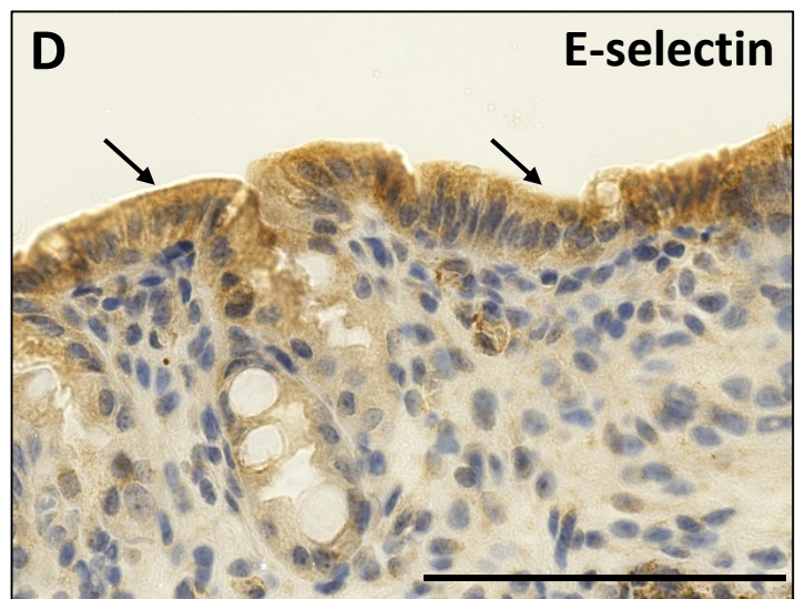
GPR4 antagonist 13
