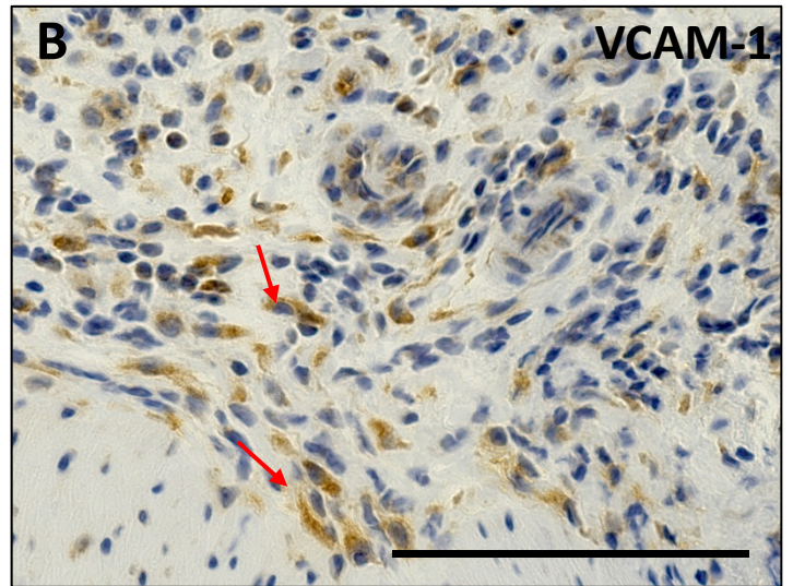
GPR4 antagonist 13
