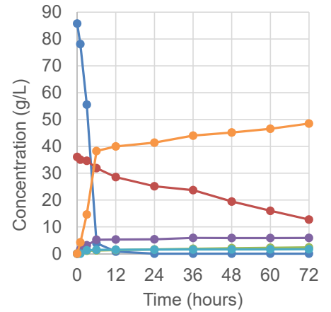
SS86 ( LpXI-T273A )
