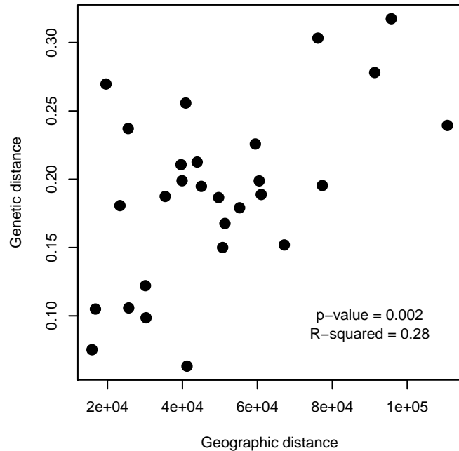
C. macromma
