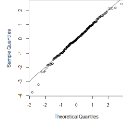
E Normal Q-Q Plot
