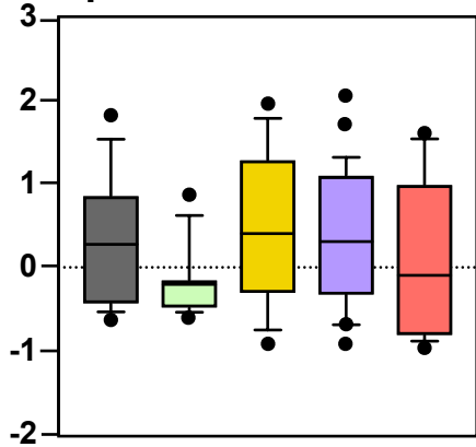
putrescine
