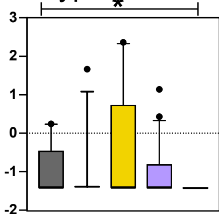
tryptamine
