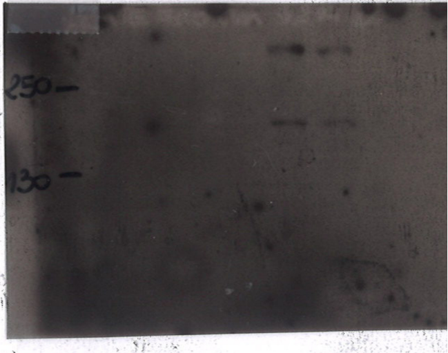
pATR-Ser428
