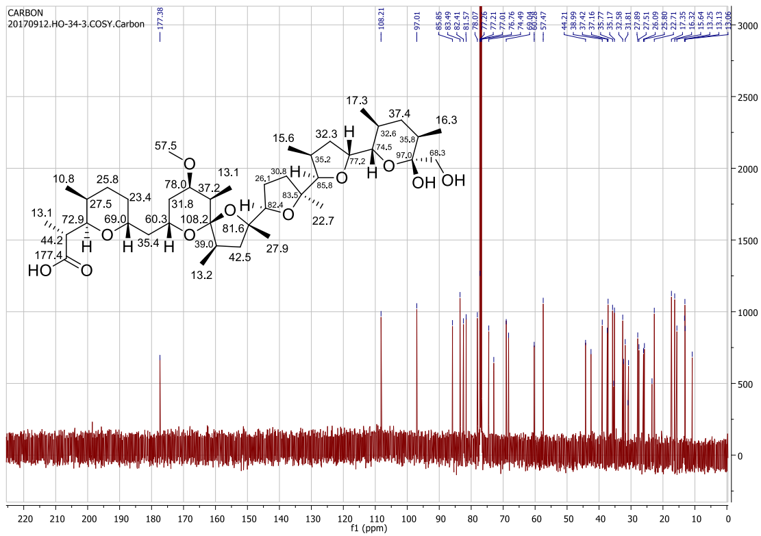
S8 Fig. ^{13}\text{C} NMR of nigericin ( 3 ) ( \text{CDCl}_3 , 125 MHz)
