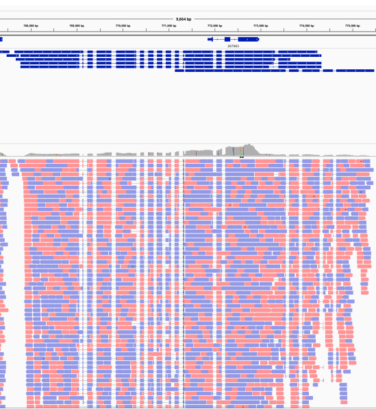
Jgi 267963
