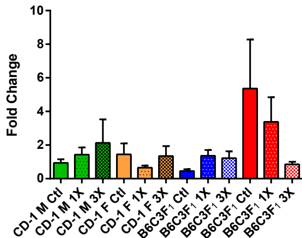
miR-29a
