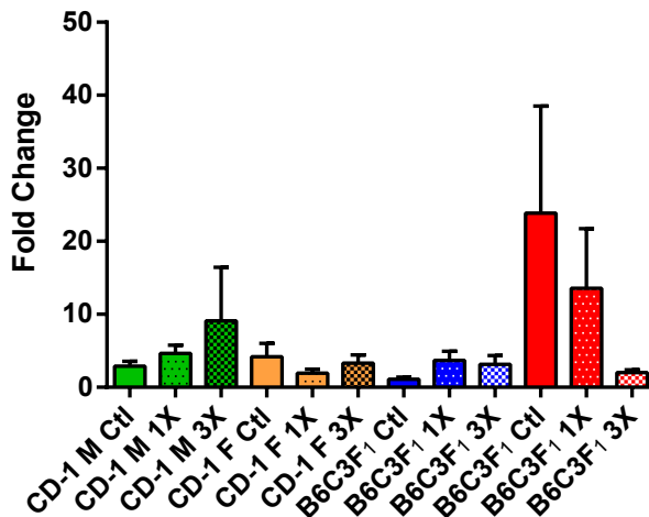
miR-101a
