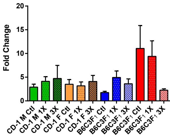
miR-122
