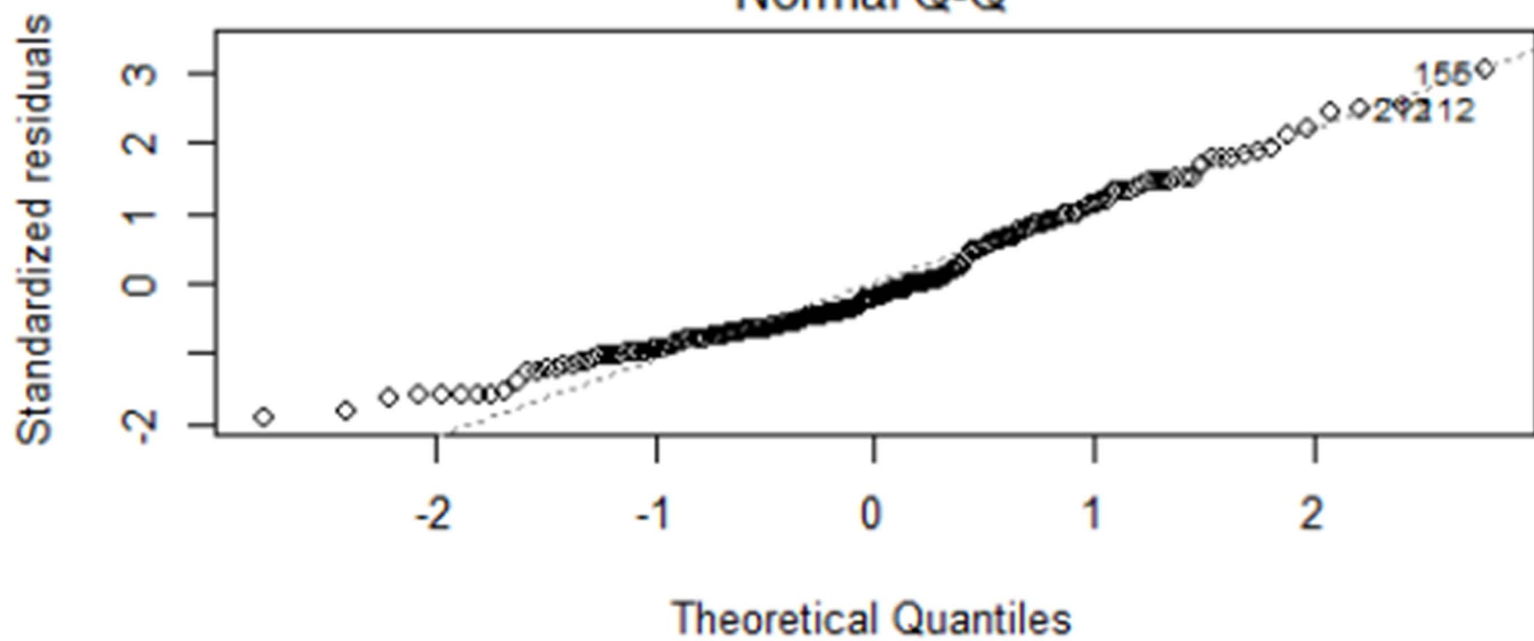
Normal Q-Q
