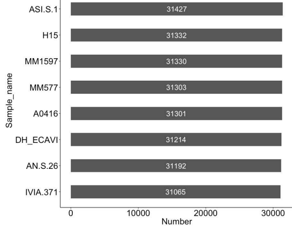
ClassII//DNA_MITE/Tc
