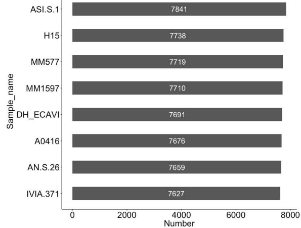
ClassII//DNA_nMITE/MuDR
