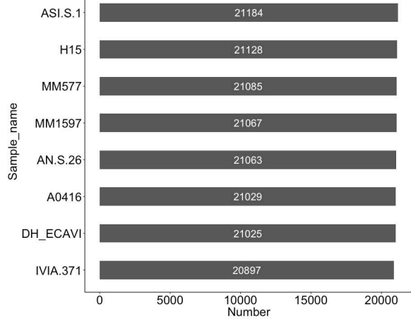
ClassII//DNA_MITE/hAT
