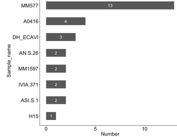
ClassII//DNA_nMITE/Harbinger
