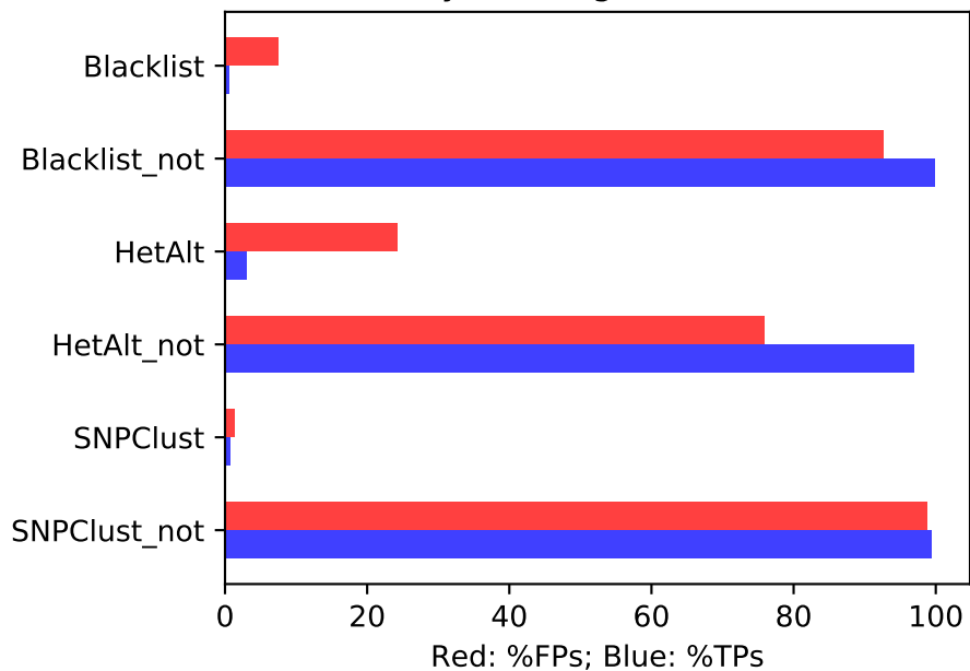
2.N.1 Binary warnings (Lab1 GIAB Indel)
