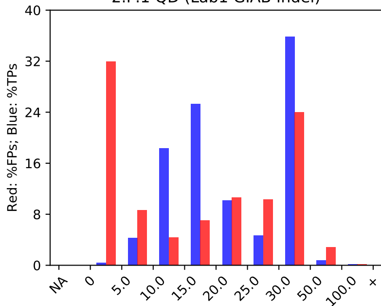
2.F.1 QD (Lab1 GIAB Indel)
