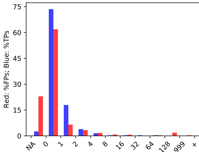
2.G.1 SB5 (Lab1 GIAB Indel)
