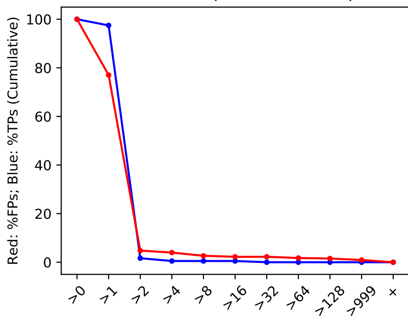
2.H.3 SB25 (Lab1 GIAB Indel)
