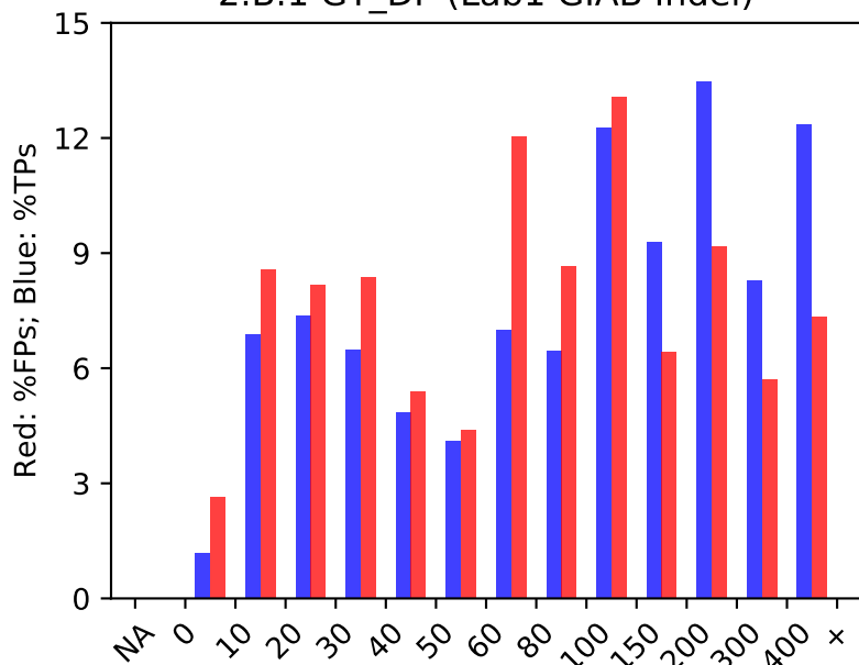
2.B.1 GT_DP (Lab1 GIAB Indel)
