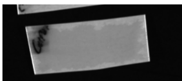
c-myc
