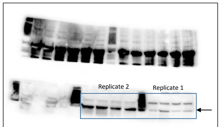
ELP3
