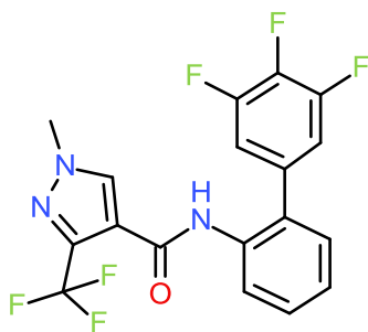
Fluxapyroxad
