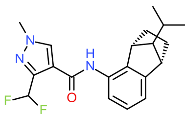
Isopyrazam
