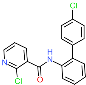
Boscalid
