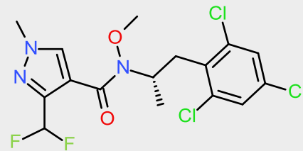
Pydiflumetofen
