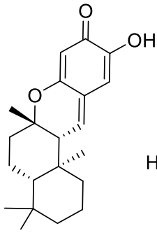
Puupehenone
