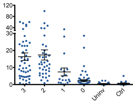
ZIC2
