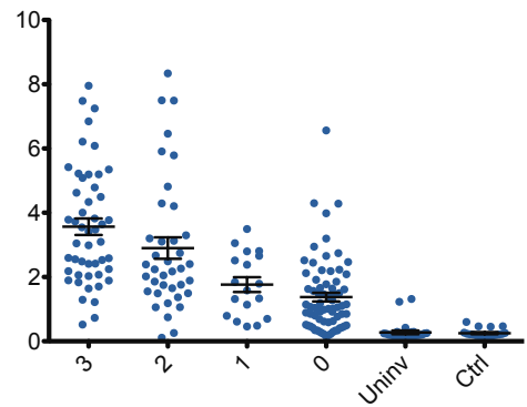
ZIC5
