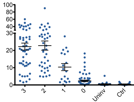
CRYBA2
