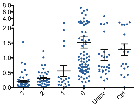
CRYBA2
