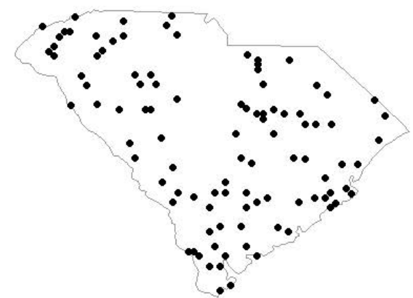
W Estimate Errors - O3
