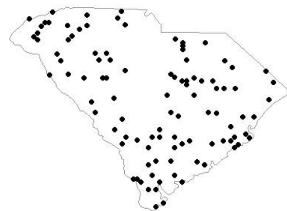
W Estimate Errors - SO4
