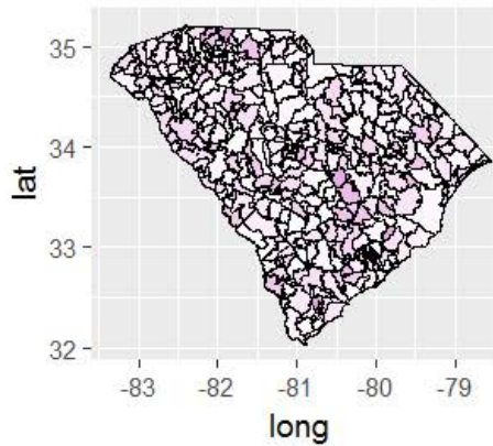
W Estimates - CO
