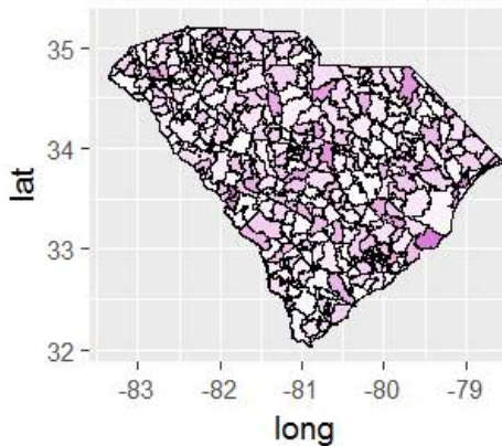
W Estimates - NH4
