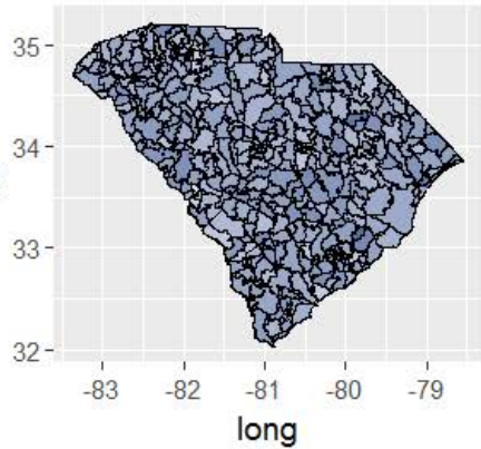
True Values - NH4
