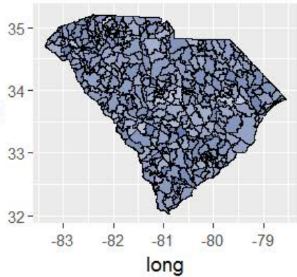
True Values - EC1
