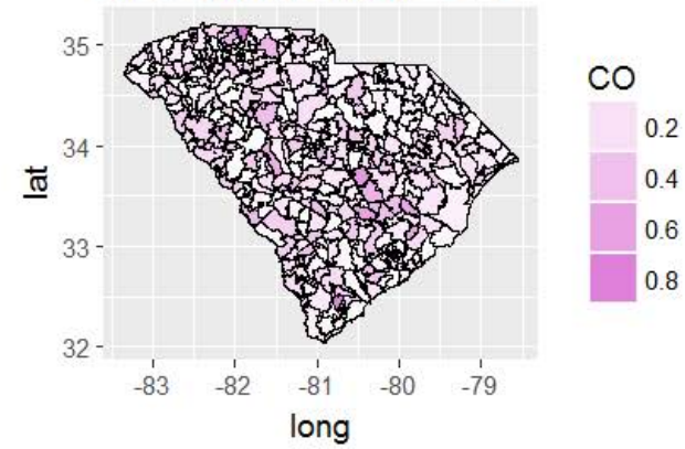
W Estimate Errors - CO
