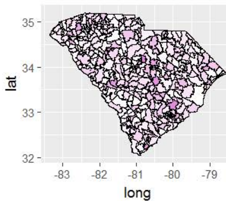
Y Estimate Errors - O3
