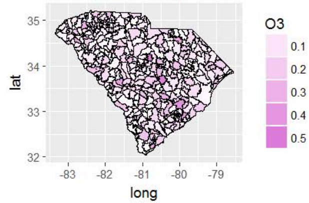
W Estimate Errors - O3
