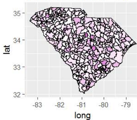
W Estimates - O3
