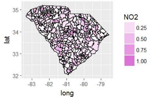
W Estimate Errors - NO2
