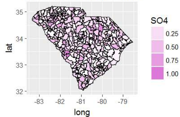
W Estimate Errors - SO4
