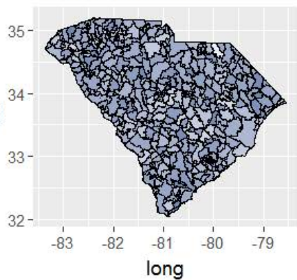
Y Estimates - O3
