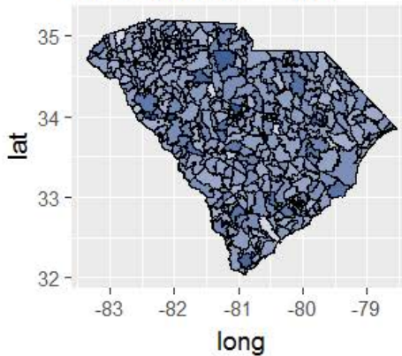
Y Estimate Errors - SO4
