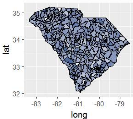
Y Estimate Errors - SO2
