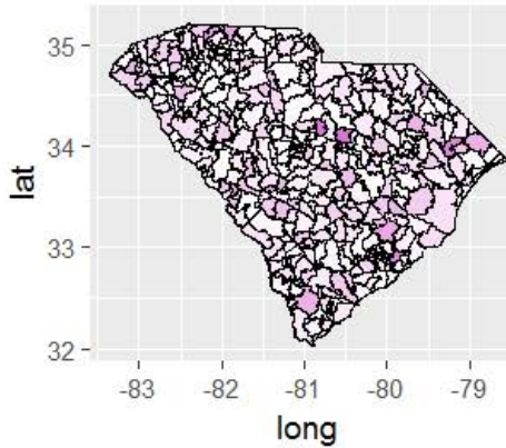
W Estimates - EC1
