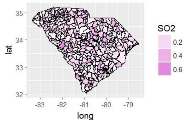
W Estimate Errors - SO2
