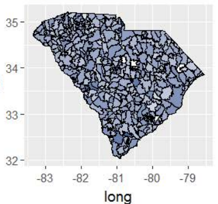
Y Estimates - EC1
