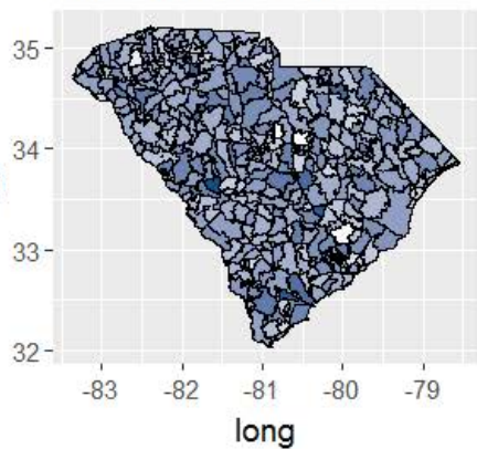
Y Estimates - O3
