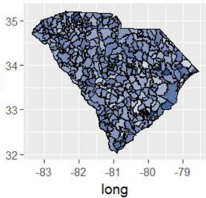
True Values - CO
