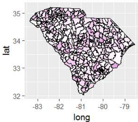
W Estimates - SO2
