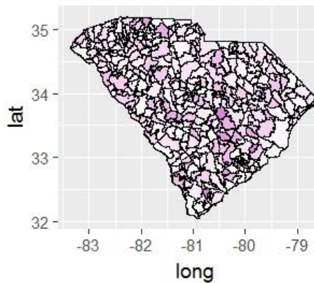
Y Estimate Errors - CO
