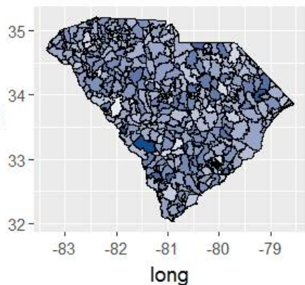
Y Estimates - SO2
