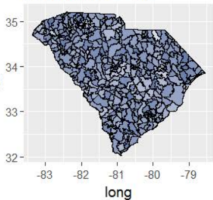
True Values - O3
