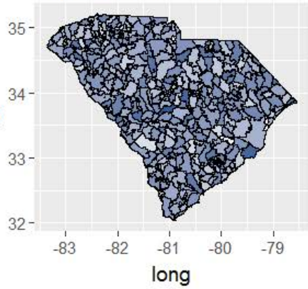
Y Estimates - NH4
