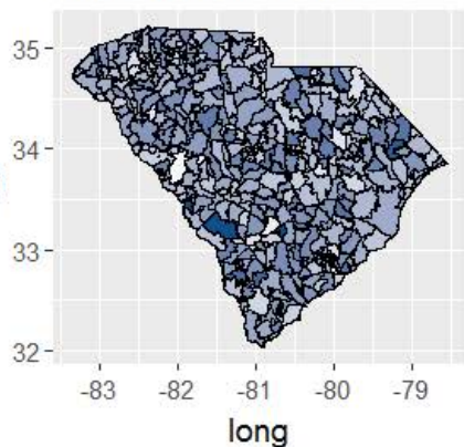
Y Estimates - SO2
