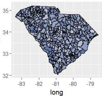
True Values - SO2
