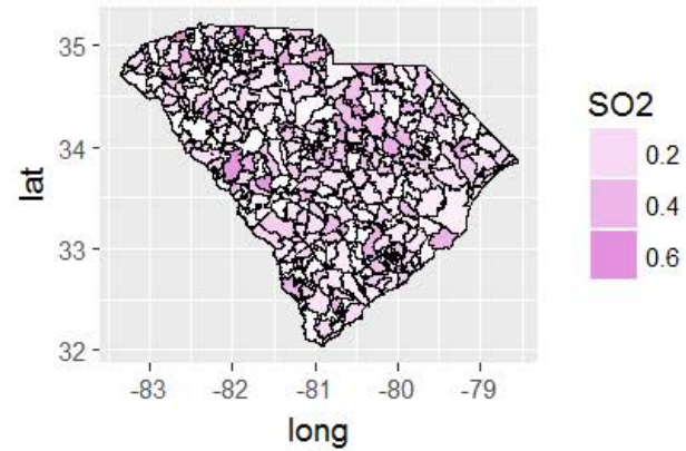
W Estimate Errors - SO2
