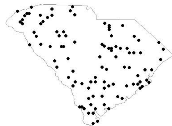
W Estimate Errors - NO2
