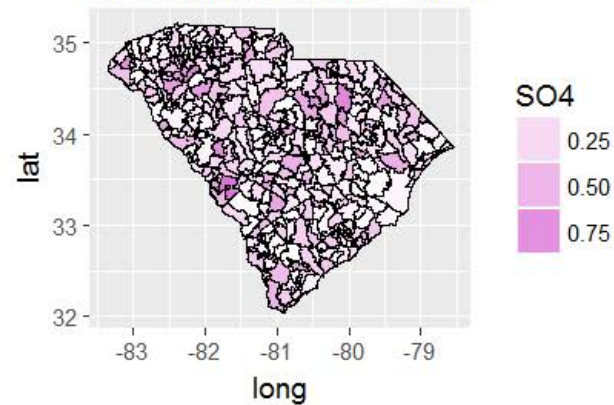
W Estimate Errors - SO4
