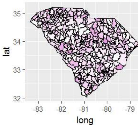
W Estimates - SO2
