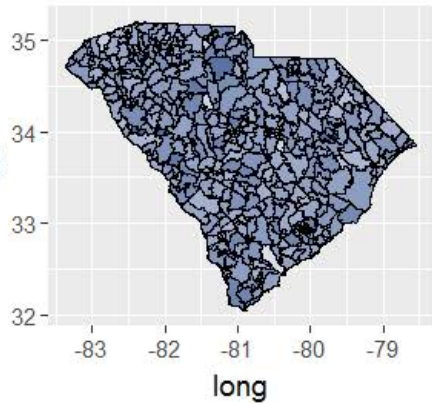
Y Estimates - SO4
