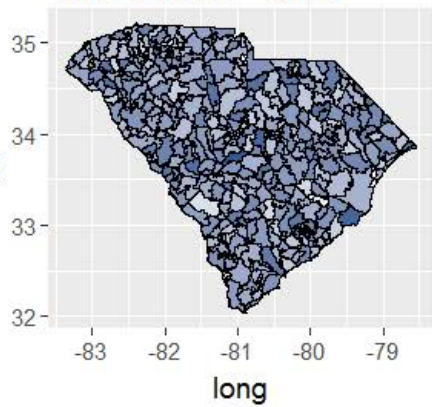
Y Estimates - NH4
