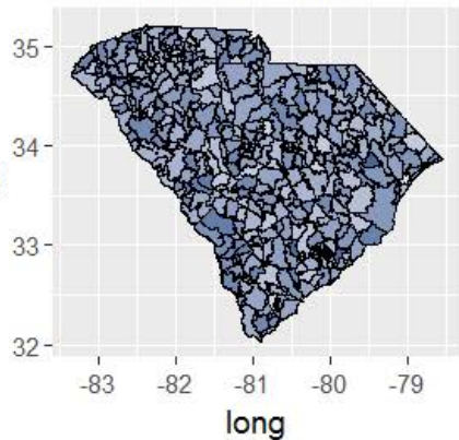
True Values - SO2
