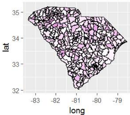
W Estimates - SO4
