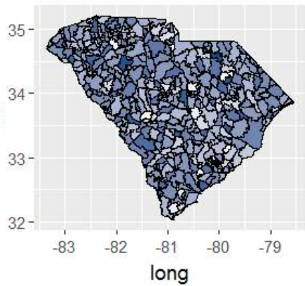
Y Estimates - NO2
