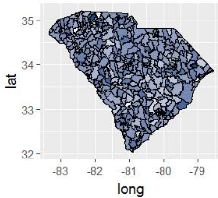
Y Estimate Errors - CO
