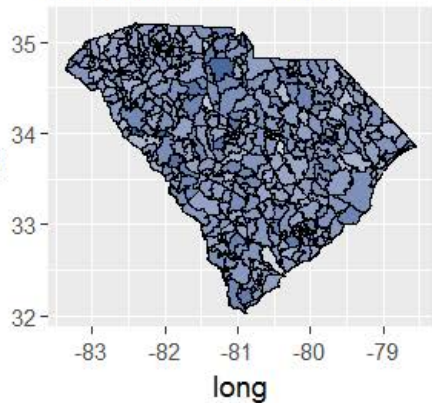
True Values - SO4
