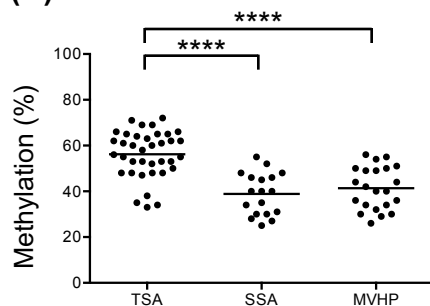
(D) SFRP2
