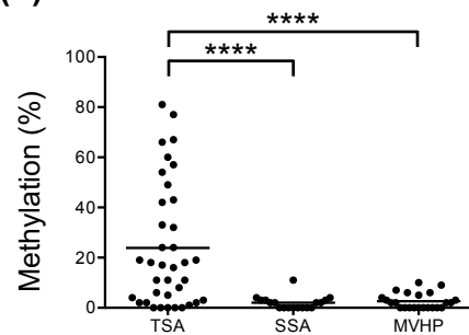
(F) SMOC1
