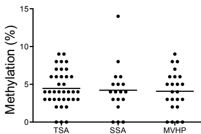
(B) MLH1
