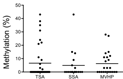
(A) CDKN2A
