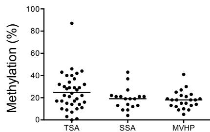
(G) GALNT14
