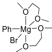
cis -PhMgBr(dme) 2 singlet
