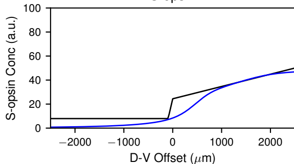
S-opsin
