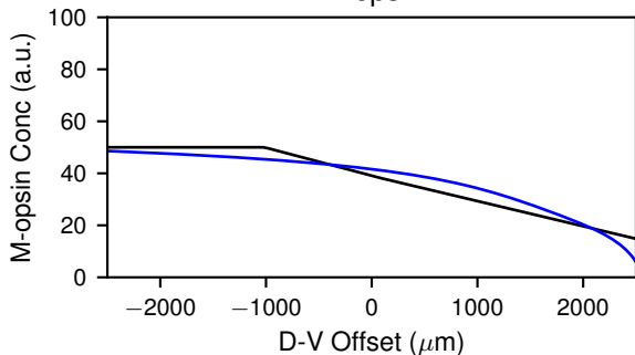
M-opsin
