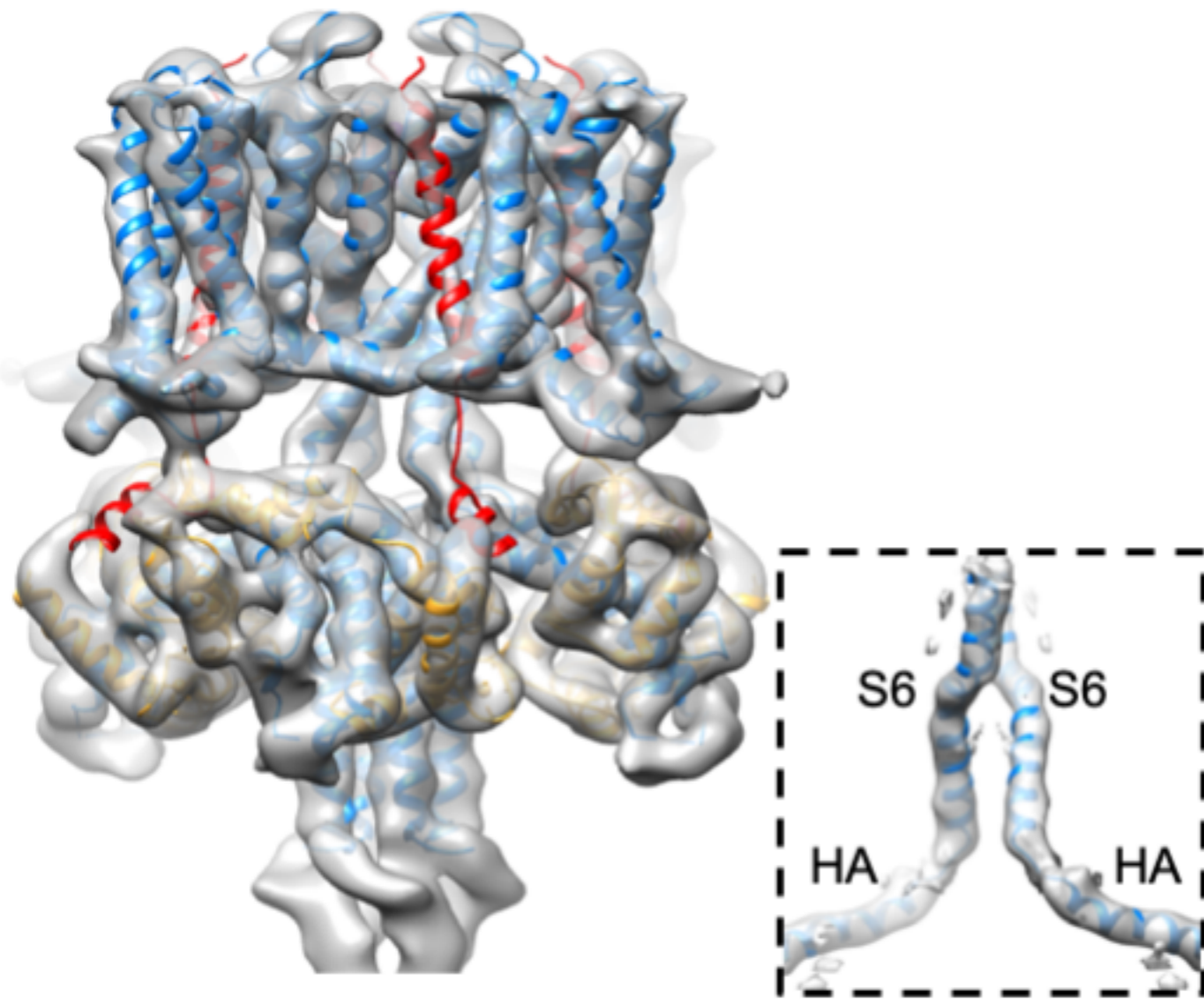
KCNQ1-KCNE3-CaM
