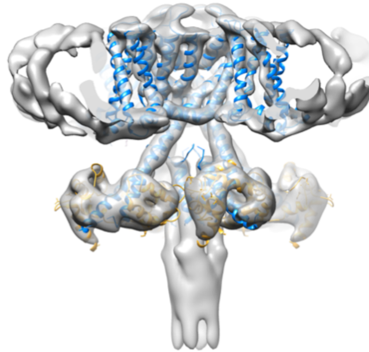
KCNQ1-CaM
