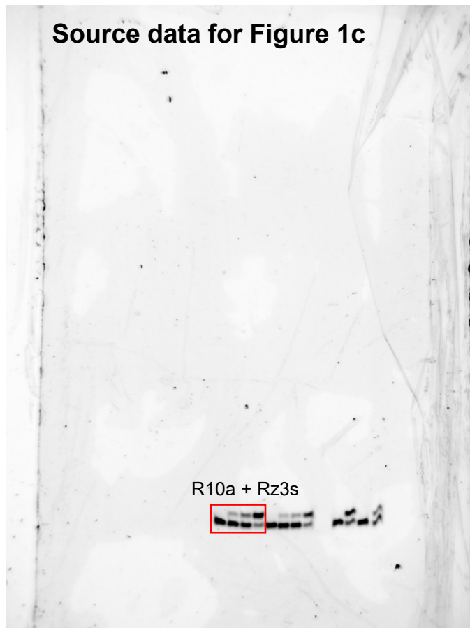
20% PAGE, 20x30 cm, 35W, 2:15 h
