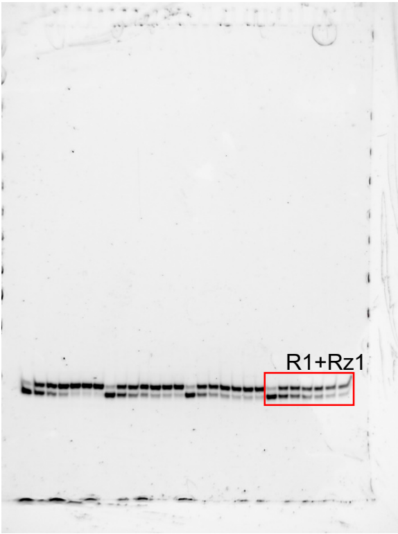
20% PAGE, 20x30 cm, 35W, 2:15 h
