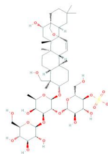
Saikosaponin 2
