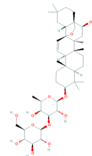
Saikosaponin E
