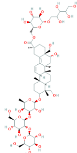
Saikosaponin U
