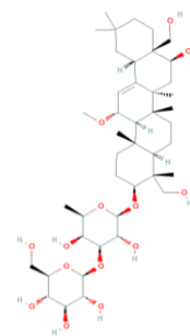
Saikosaponin B3
