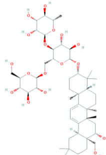
Saikosaponin I
