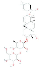
Saikosaponin D
