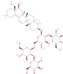
Saikosaponin Q
