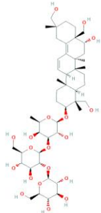
Saikosaponin R
