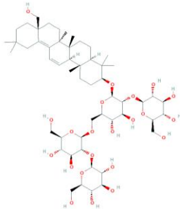
Saikosaponin K
