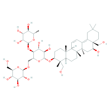
Saikosaponin N
