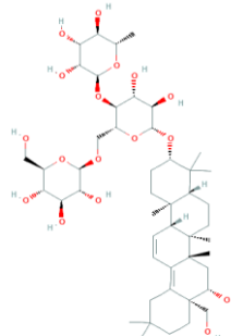
Saikosaponin H
