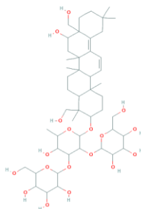
Saikosaponin 1b
