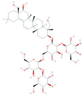
Saikosaponin O
