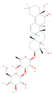
Saikosaponin B2
