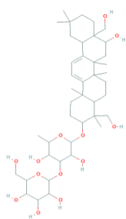
Saikosaponin G
