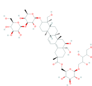
Saikosaponin V
