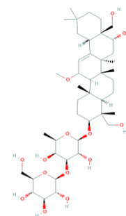
Saikosaponin E
