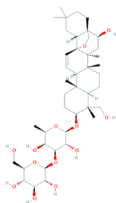
Saikosaponin A
