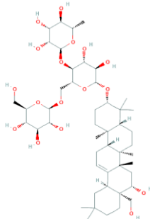
Saikosaponin F
