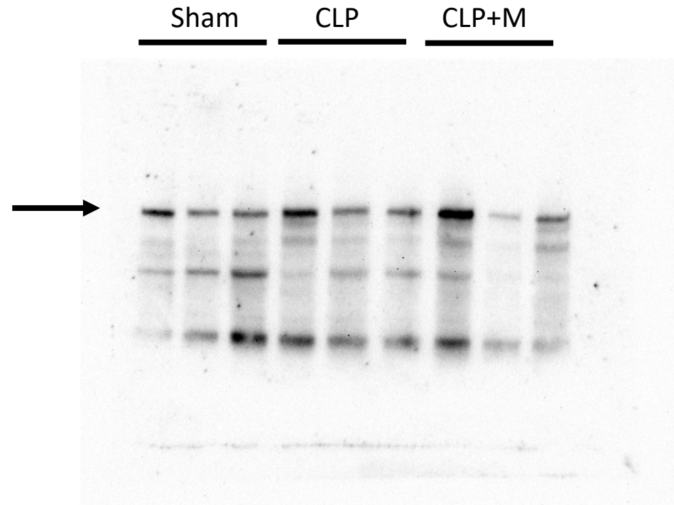
Caspase 1 Blot
