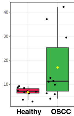
PC 17:0;0_20:4;0
