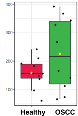
PC 18:0;0_18:2;0
