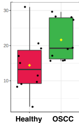
PC 17:1;0_18:1;0
