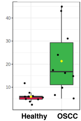
PC 16:1;0_20:4;0
