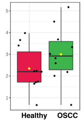
PC 17:1;0_18:0;0
