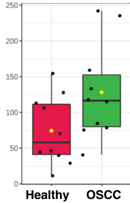
PC 16:1;0_18:1;0
