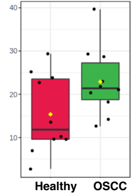
PC 16:1;0_18:0;0
