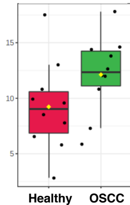
PC 17:1;0_18:2;0
