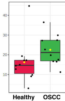
PC 17:0;0_18:1;0
