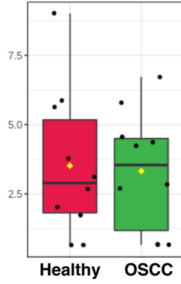
PC 16:1;0_17:0;0
