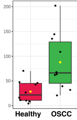
PC 16:1;0_16:1;0
