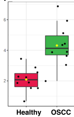
PC 16:1;0_20:3;0
