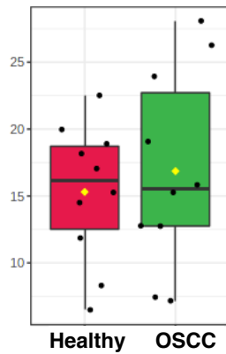
PC 17:0;0_18:2;0
