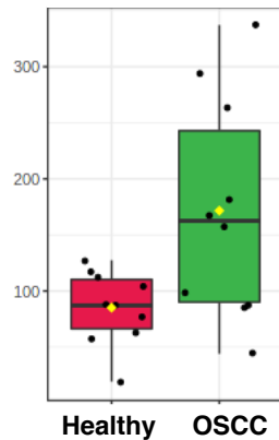
PC 18:0;0_18:1;0
