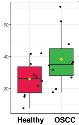
PC 16:1;0_18:2;0
