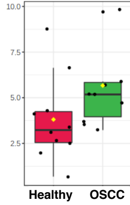
PC 16:1;0_17:1;0
