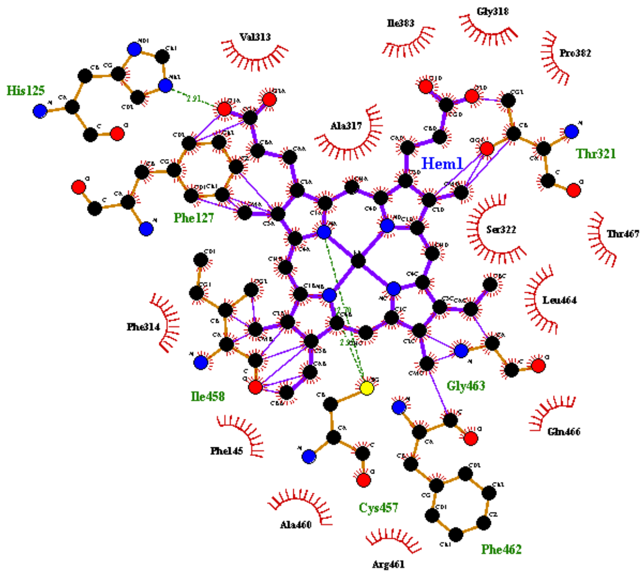
CYP6BK3_q1 BD TEPP
