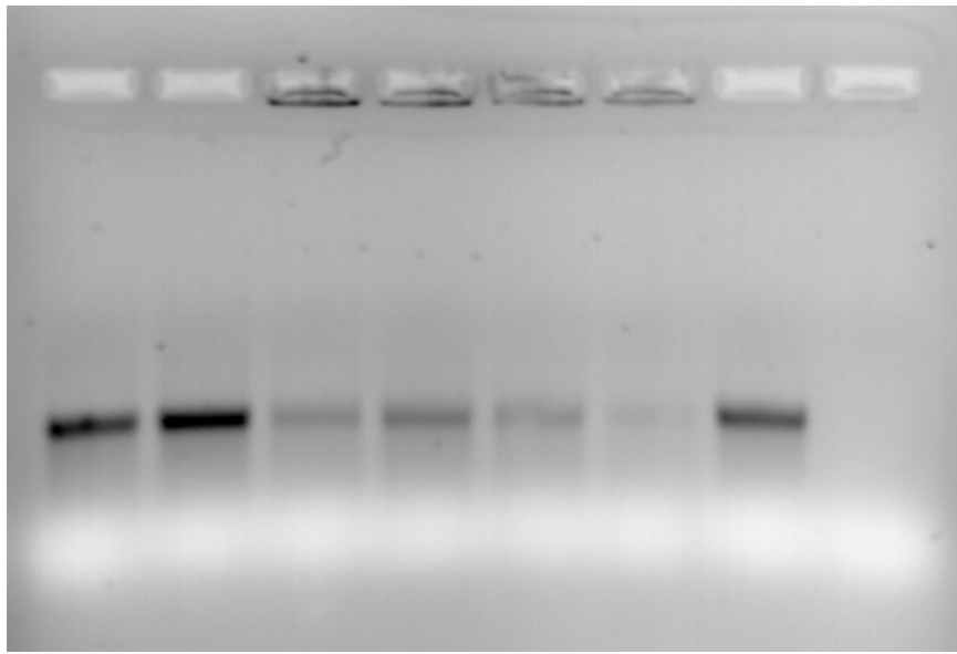
sigF
