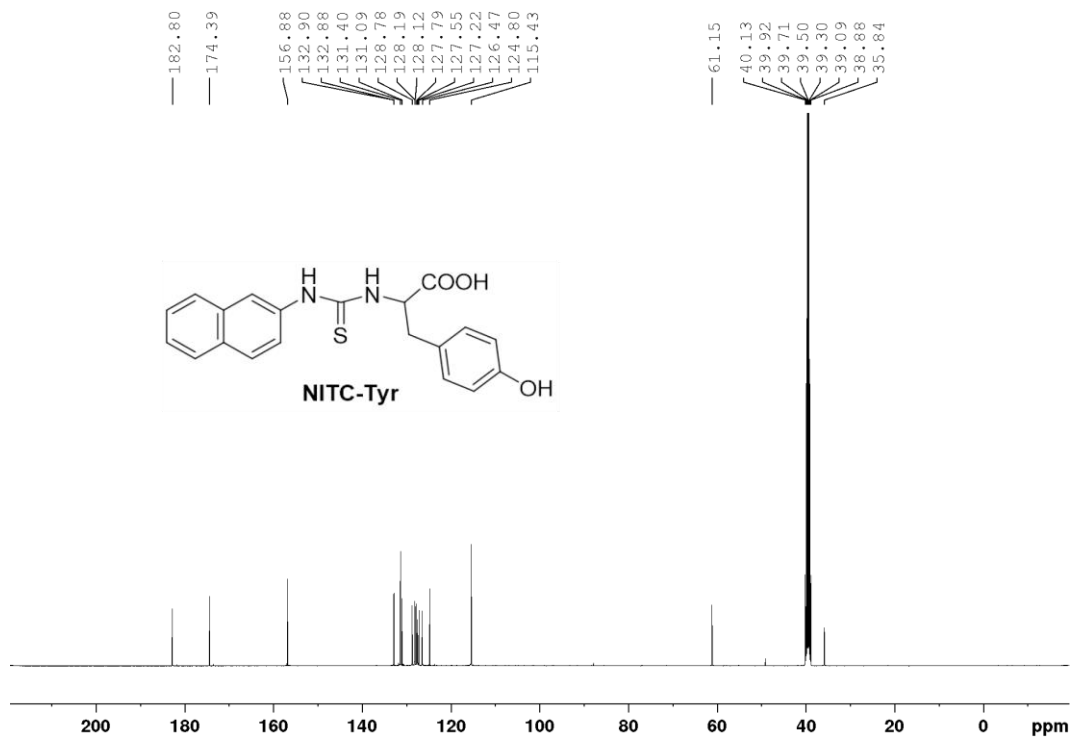
Fig. S33 13 C NMR spectrum of NITC-Tyr.
