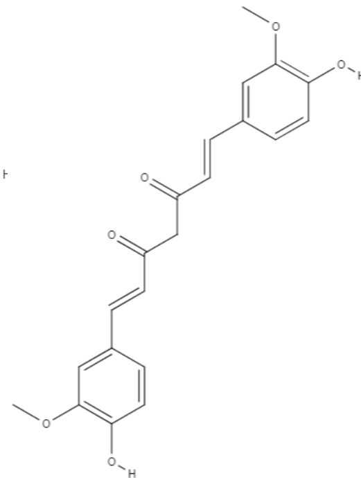
Curcumin
