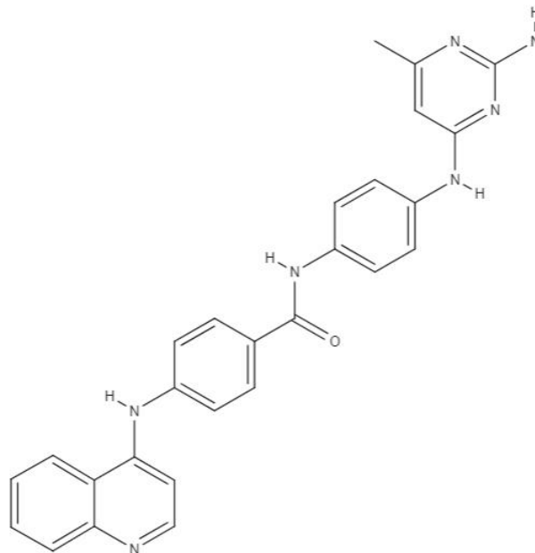
SGI-1027
