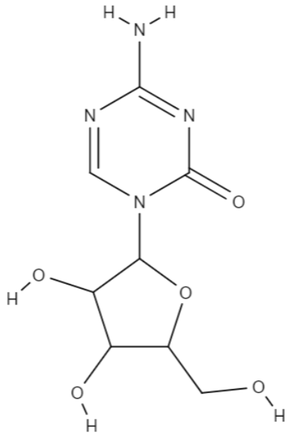
5-azacytidine (5-aza)
