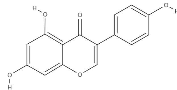
Genistein
