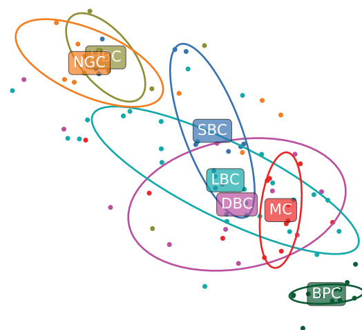
V1 Layer 4
