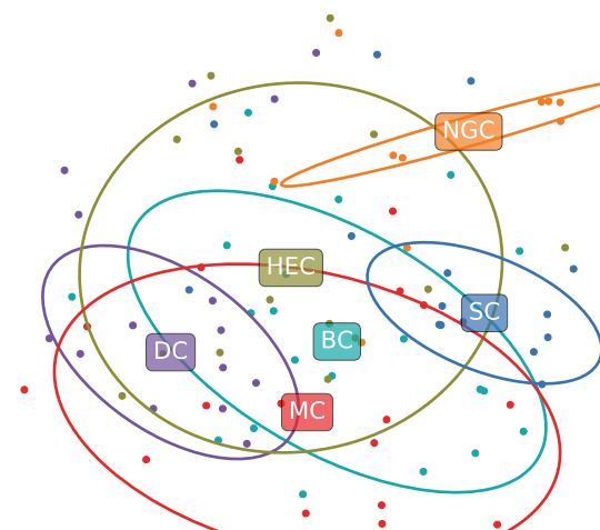
V1 Layer 5
