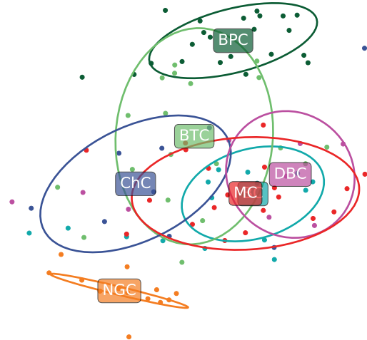
V1 Layer 2/3
