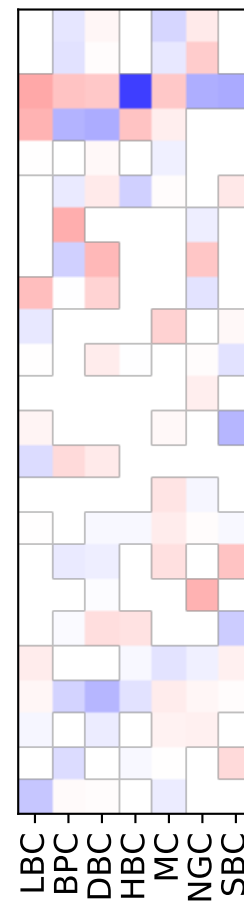
V1 Layer 4
