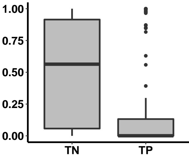
pRec p = 5e-21
