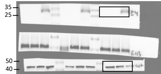
E4orf6: input hnRNP-C2
