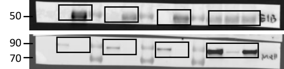
E1B55K: HeLa | U2OS | A549 | HEK293
