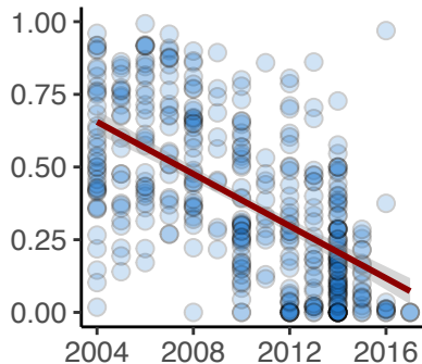
pfmdr1 86Y
