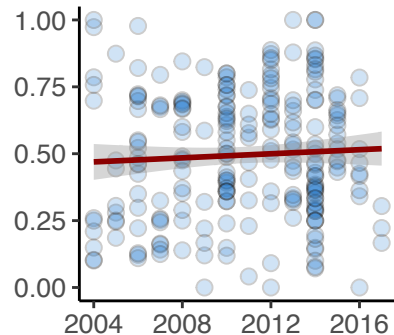
pfmdr1 184F
