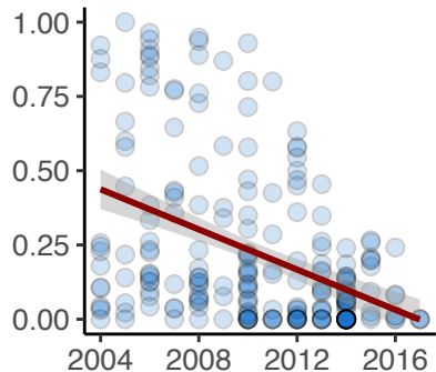
pfmdr1 1246Y
