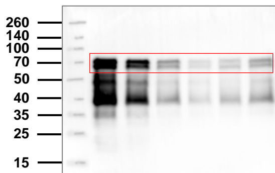
YAP1
