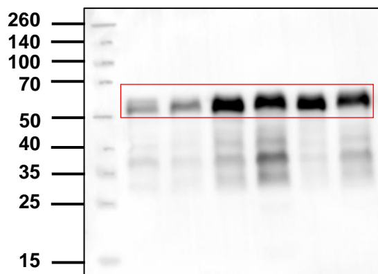
WWTR1
