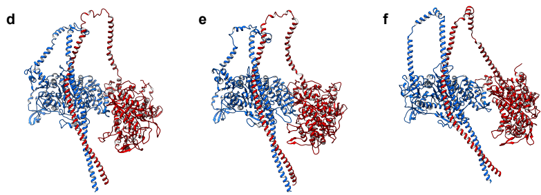
d Cardiac IHM model - 5TBY e Cardiac IHM model - MS01 f Cardiac IHM model - Robert-Paganin et al., (2018) (SD2)
