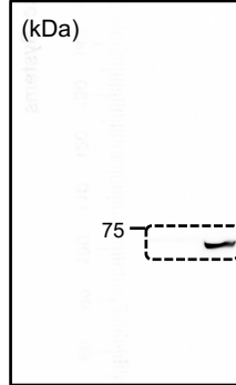
Blot: anti-mitHSP70
