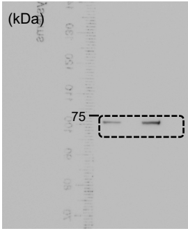
Blot: anti-NCOA4
