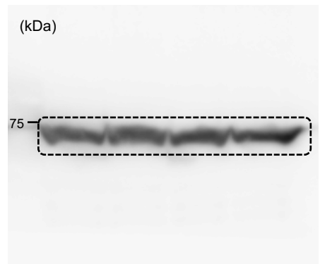
Blot: anti-mitHSP70
