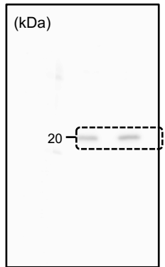
Blot: Tom20
