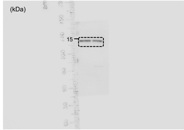
Blot: anti-VDAC
