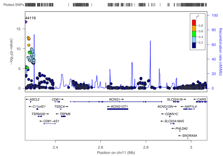
(b) PrCa p-values
